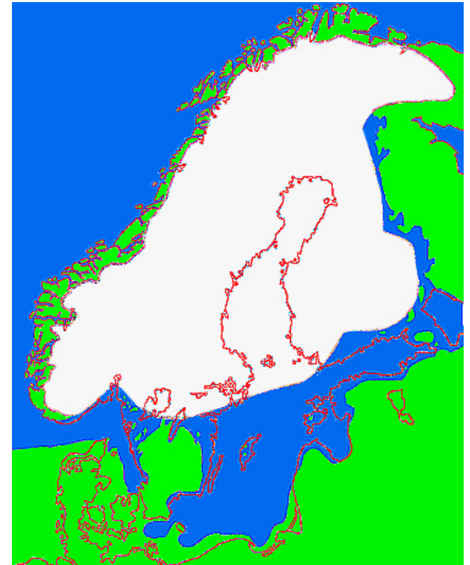
KUVA 1. Jääpeitteen laajuus noin 8 000 eKr.
